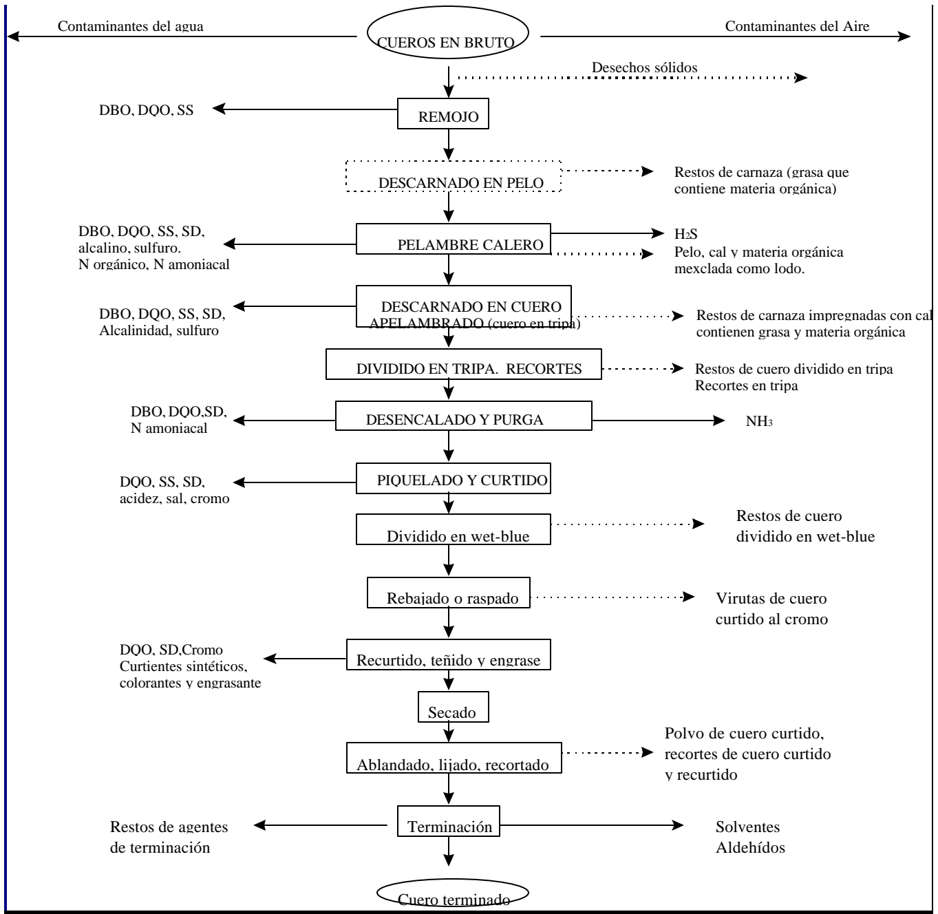
Figura N°1: Esquema proceso de producción cueros curtidos
