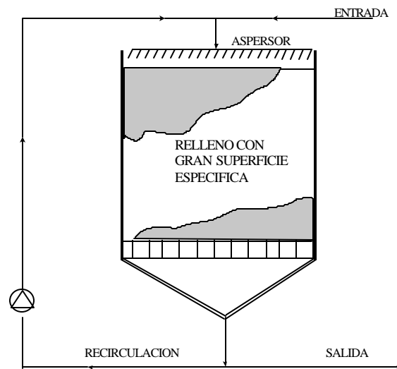
Figura N°3: Esquema de un filtro percolador
